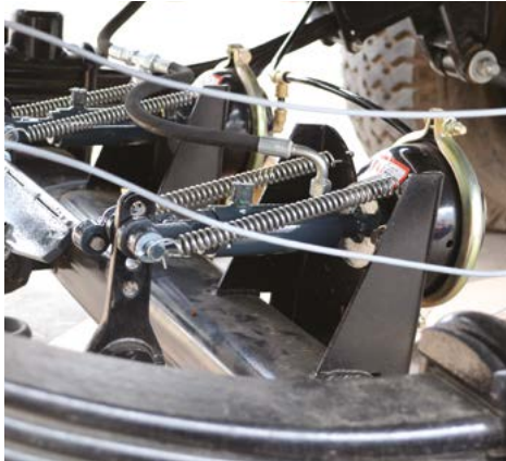
Комбінована гальмівна система
