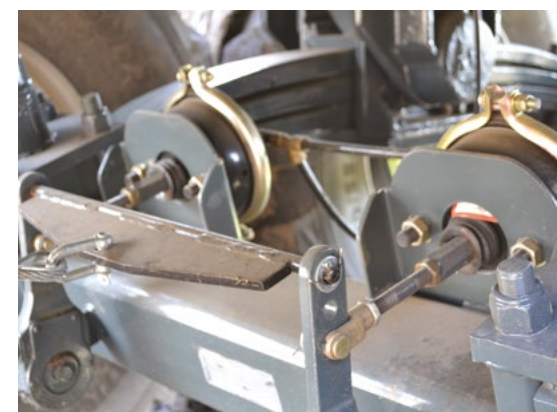
Пневматическая тормозная система
