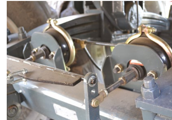
Ваздушни кочioni систем
