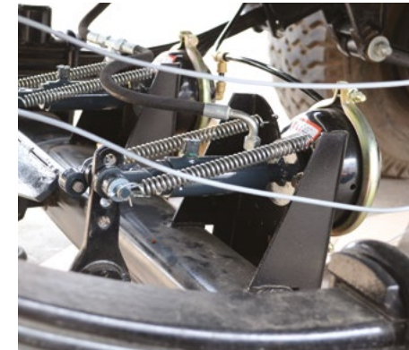
Комбиновани кочioni систем
