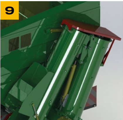
ЗАШТИТНИ ПОКЛОПАЦ СВРДЛА ОД ПАДАВИНА
