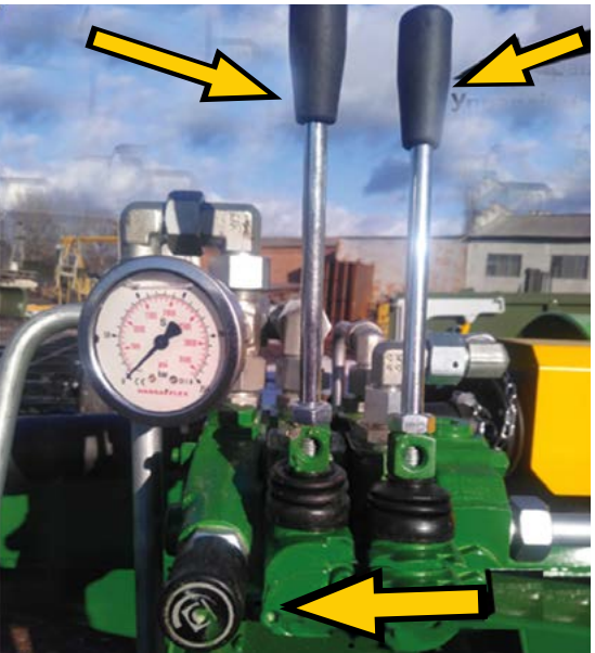
Rankovės vyniojimo greičio reguliatorius
