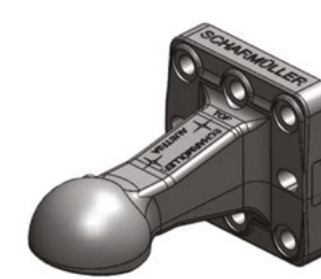
Koule Ø80
