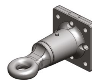
Otočné oko Ø50
