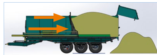
La metà del fondo si muove con la parete anteriore
