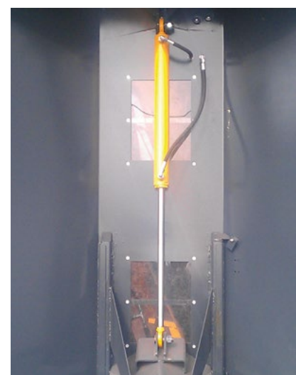
Sportello di chiusura idraulica per coclea grano
