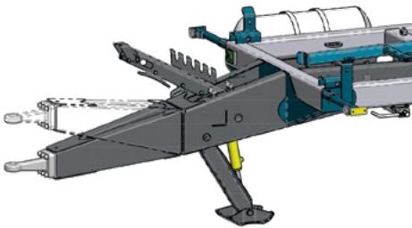
Kallutatav haakekonks
