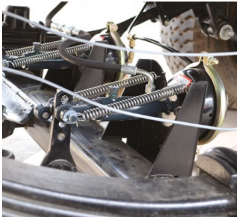
Kombineeritud pidurisüsteem.
