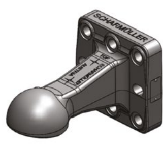
hemisphere Ø80
